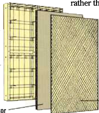
RP Prefilter
